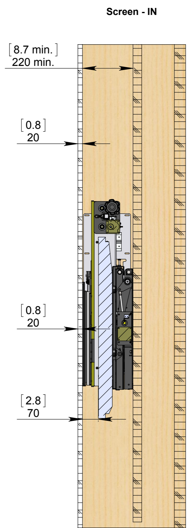
SECTION A-A SCALE 1 : 10
