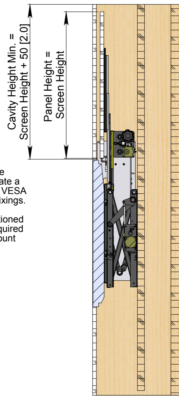
SECTION D-D SCALE 1 : 12
