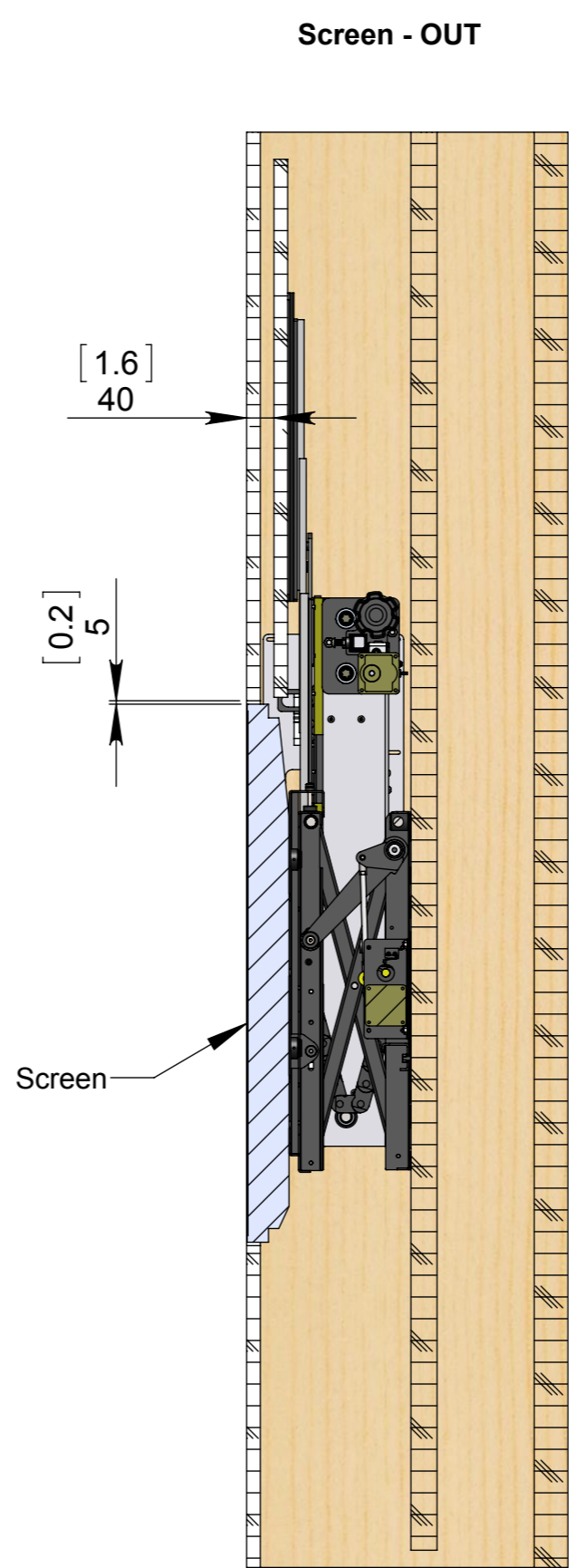
SECTION B-B SCALE 1 : 10
